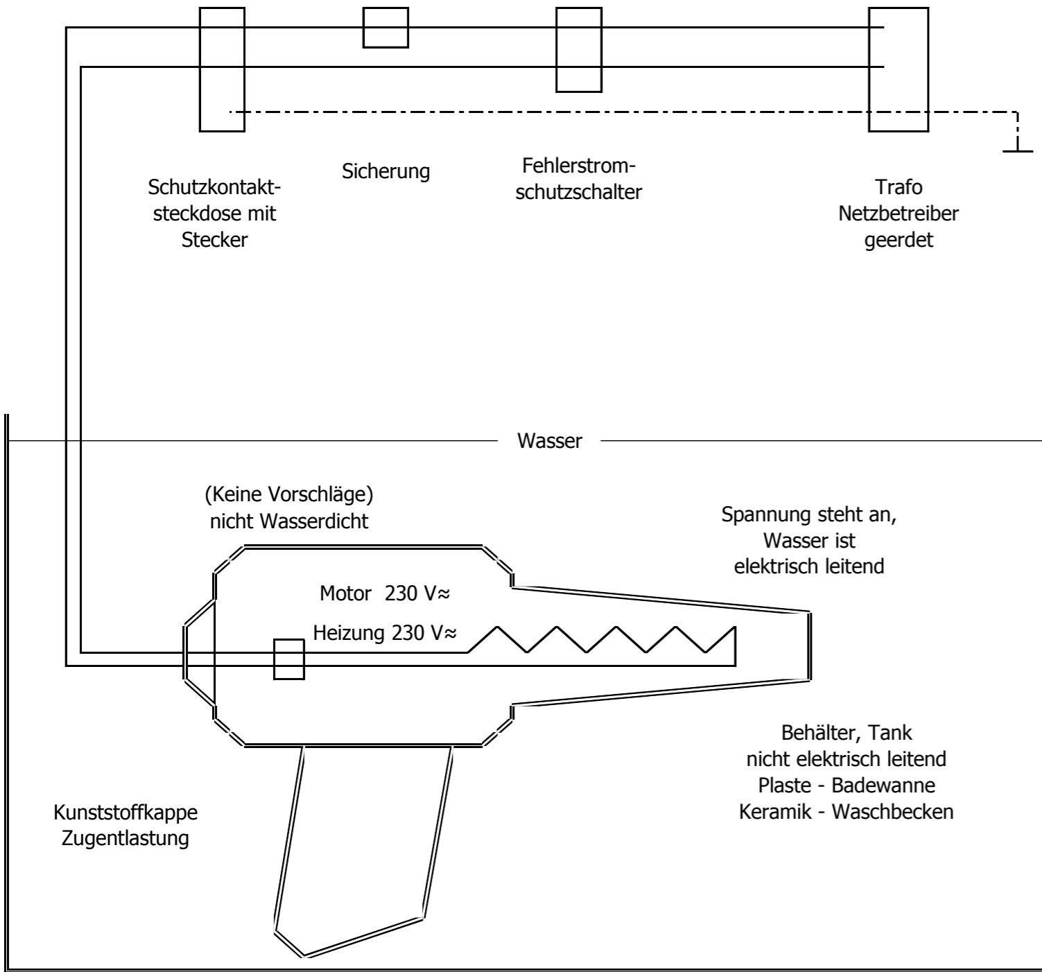
Stand der Technik, ohne Schutzleiter
