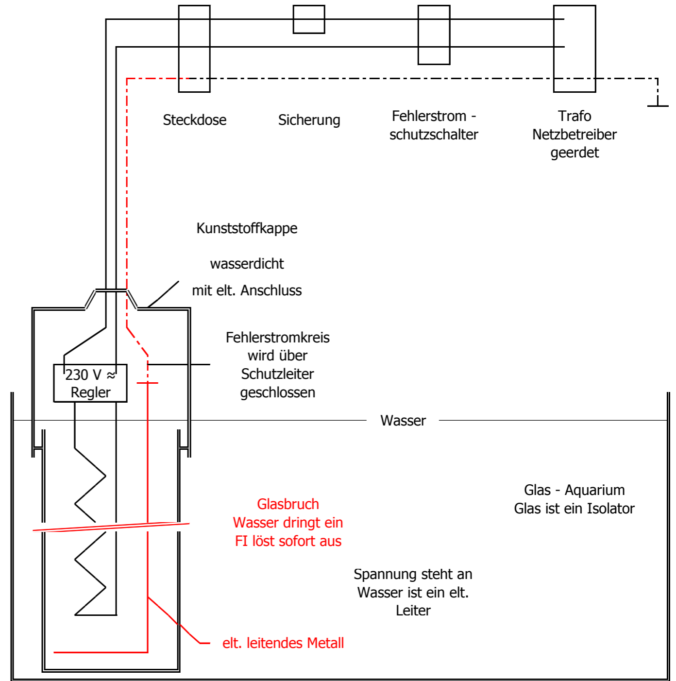
meine Erfindung, mit Schutzleiter
